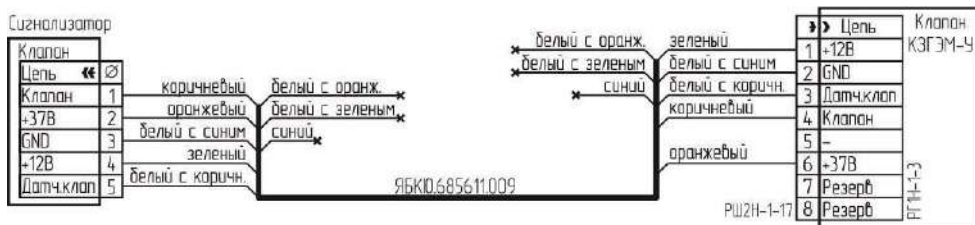
Рисунок В.3 – Схема подключения клапана КЗГЭМ-У с разъемом P11H-1-3.
